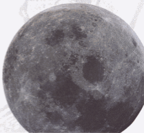
Кратеры на поверхности Луны
