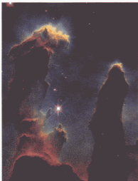
Телескоп Хаббла позволила отчетливо увидеть небесные тела, что прежде было невозможно из-за искажений в атмосфере Земли
