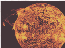
Ядерные взрывы на поверхности Солнца
