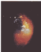
Изображение соседних и дальних галактик в телескопе Хаббла. Ночное небо всегда притягивало человека
